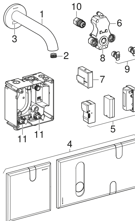
Kuva 2: Geberit-pesuallashanat Piave ja Brenta, seinäasennus
