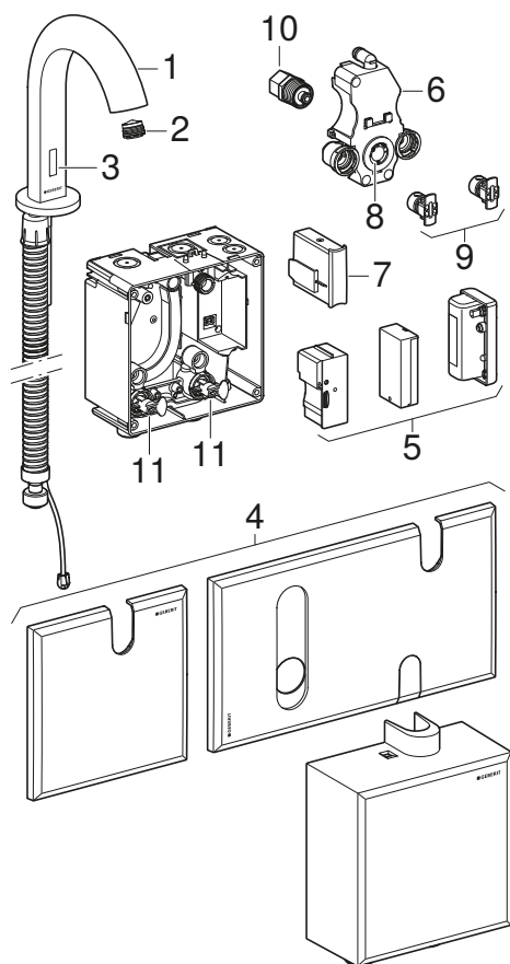
Abbildung 1: Geberit Waschtischarmaturen Piave und Brenta, Standmontage
