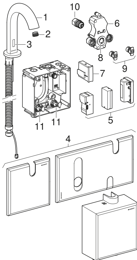
Slika 1: Umivalniške armature Geberit Piave in Brenta, stoječa montaža
