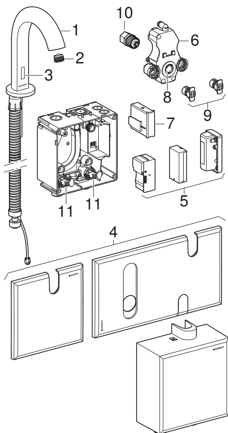
Obrázok 1: Umývadlové armatúry Geberit Piave a Brenta, stojaca montáž
