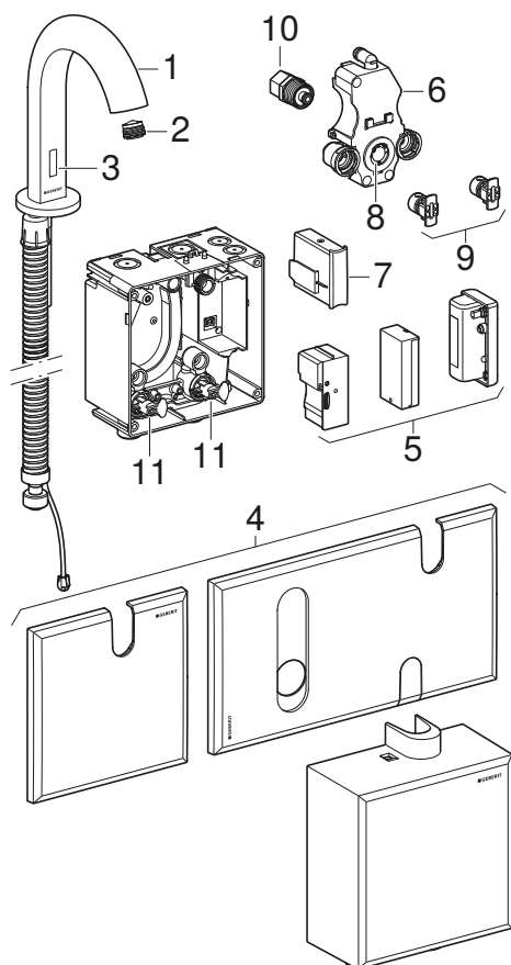
Joonis 1: Ettevõtte Geberit valamusegistid Piave ja Brenta, seisvad
