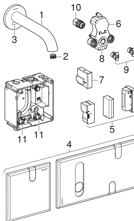
Billede 2: Geberit håndvaskarmaturer Piave og Brenta, vægmontage
