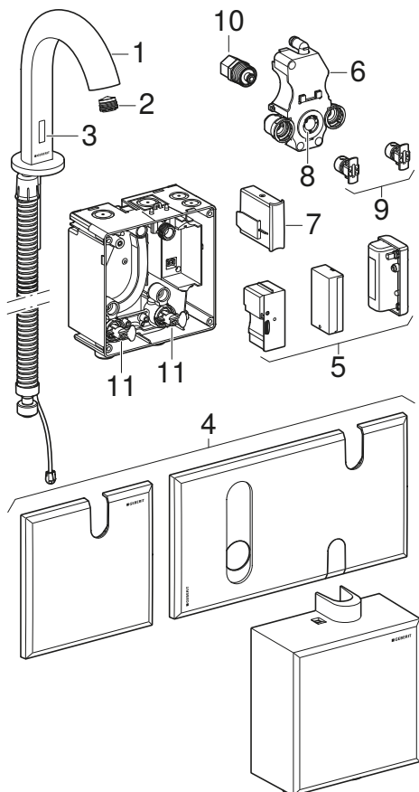
1 Paveikslas: Geberit praustuvų maišytuvai Piave ir Brenta, montuojami prie stovo
