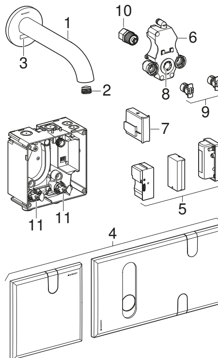
Mynd 2: Geberit handlaugatæki Piave og Brenta, veggfest
