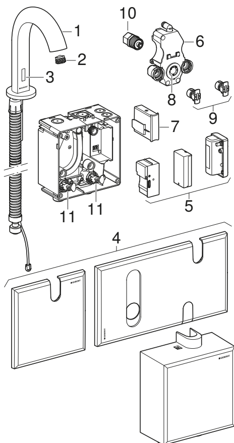
Figura 1: Rubinetterie per lavabo Geberit Piave e Brenta, montaggio a pianale
