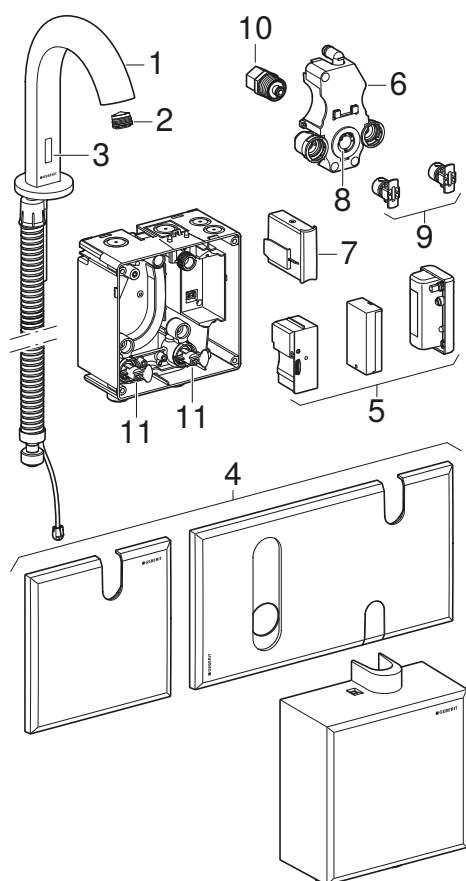
Slika 1: Geberit armature za umivaonik Piave i Brenta, stojeća montaža
