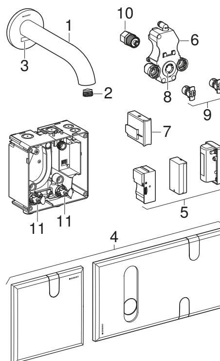
Obrázek 2: Umyvadlové armatury Geberit Piave a Brenta, nástěnná montáž
