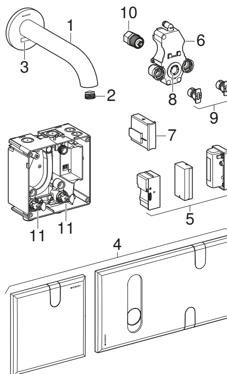
Rysunek 2: Baterie umywalkowe Geberit Piave i Brenta, montaż naścienny
