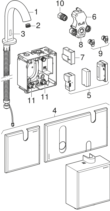
Şekil 1: Geberit lavabo bataryaları Piave ve Brenta, ankastre montaj
