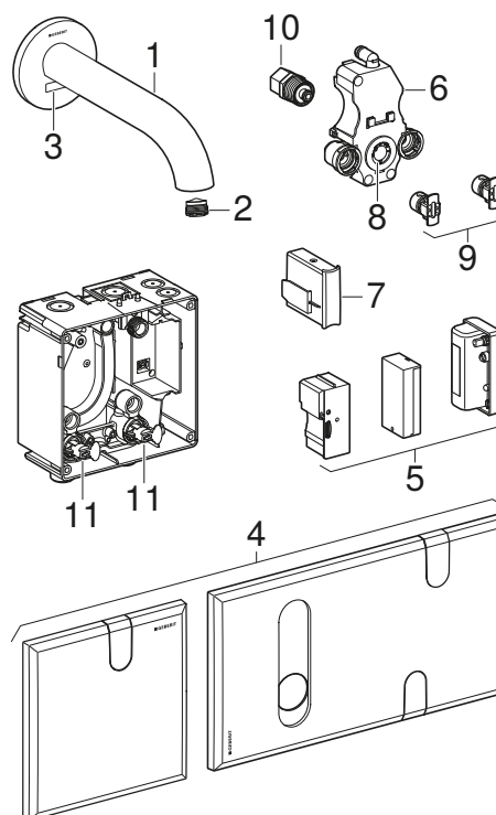
Figura 2: Grifos electrónicos para lavabos Geberit Piave y Brenta, montaje suspendido
