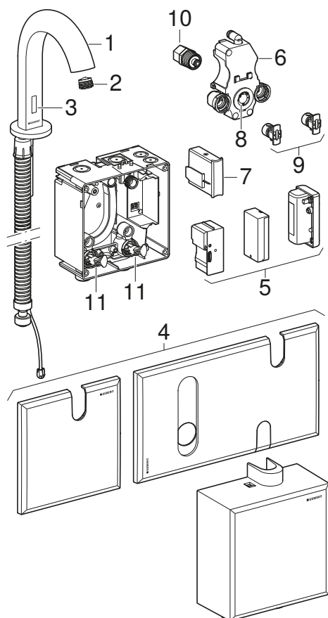
Rysunek 1: Baterie umywalkowe Geberit Piave i Brenta, stojące
