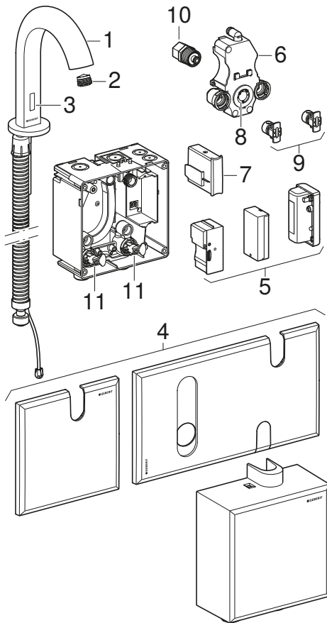
Figura 1: Armături pentru chiuvetă Geberit Piave și Brenta, montaj fix
