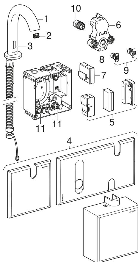
Obrázek 1: Umyvadlové armatury Geberit Piave a Brenta, stojací montáž
