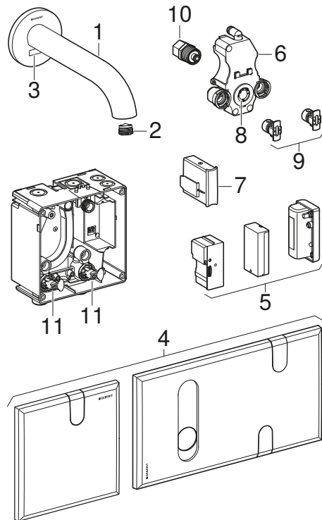
插图 2: Geberit 盥洗台感应龙头 Piave 和 Brenta, 壁挂式安装
