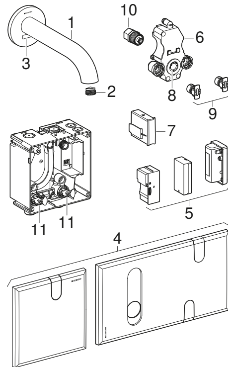
Figura 2: Armături pentru chiuvetă Geberit Piave și Brenta, montaj mural
