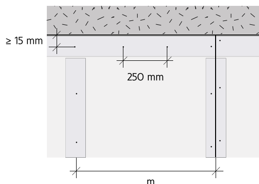
Figura 103: Aparafusamento das placas aos perfis de topo.
