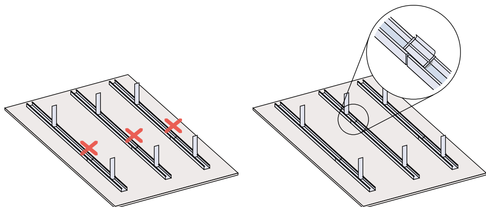
Figura 156: Desfasamento de emendas em perfis.
