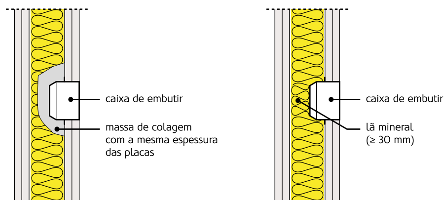
Figura 44: Isolamento de aberturas para aplicação de caixas técnicas.
