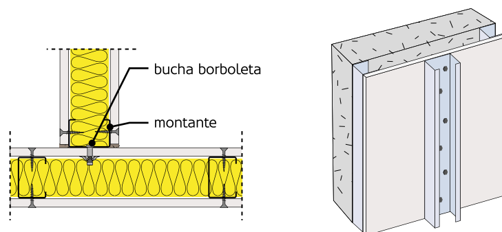
Figura 74: Ligação de um perfil montante de arranque a um sistema existente.
