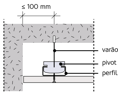
Figura 154: Distância dos perfis da estrutura portante relativamente às paredes periféricas.
