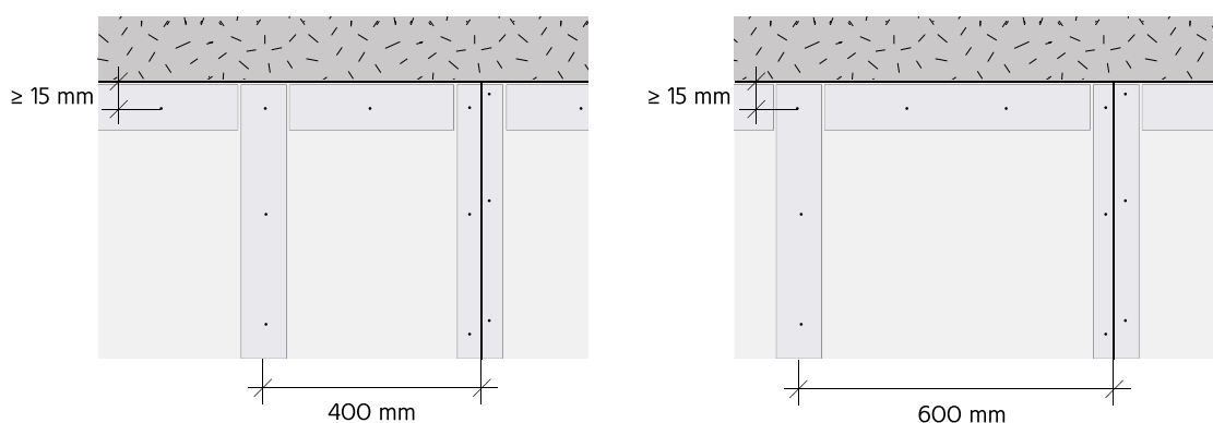
Figura 102: Aparafusamento das placas aos perfis de topo.
