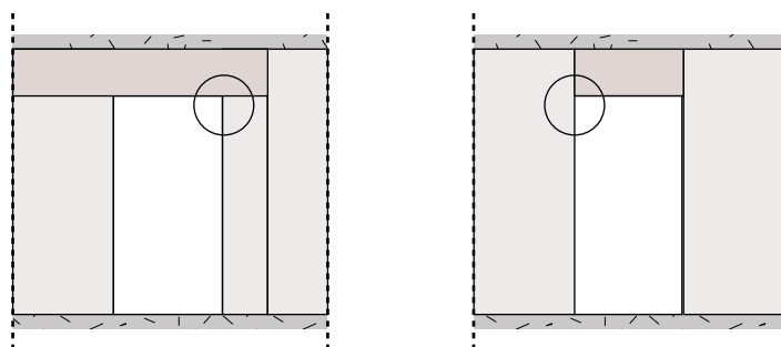
Figura 94: Contorno de vãos em revestimentos diretos com cola adesiva.
