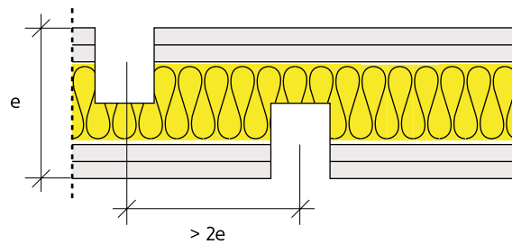
Figura 46: Desfasamento de elementos embutidos.
