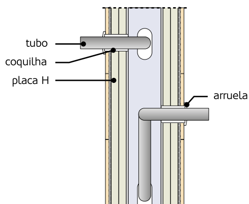
Figura 45: Selagem de aberturas para passagem de tubagem de água.
