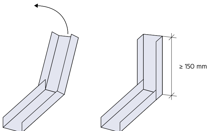
Figura 59: Quinagem dos perfis raia em zonas de aberturas.
