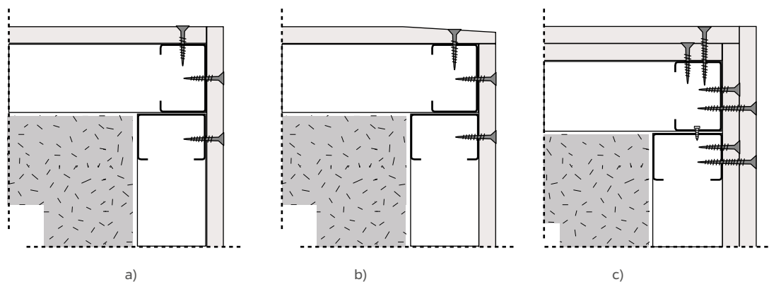
Figura 126: Ligações em cantos salientes:
