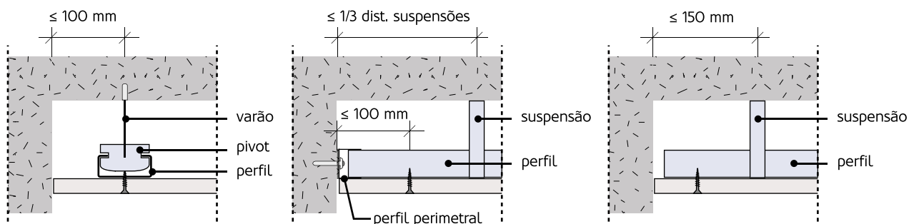
Figura 150: Distância dos pendurais e suspensões relativamente às paredes periféricas.
