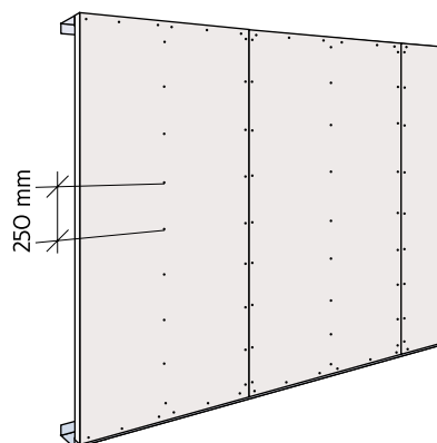
Figura 81: Afastamento entre fixações das placas aos perfis montante.
