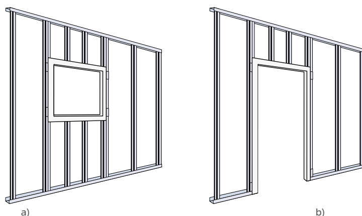
Figura 76: Estrutura metálica em: a) janelas; b) portas.
