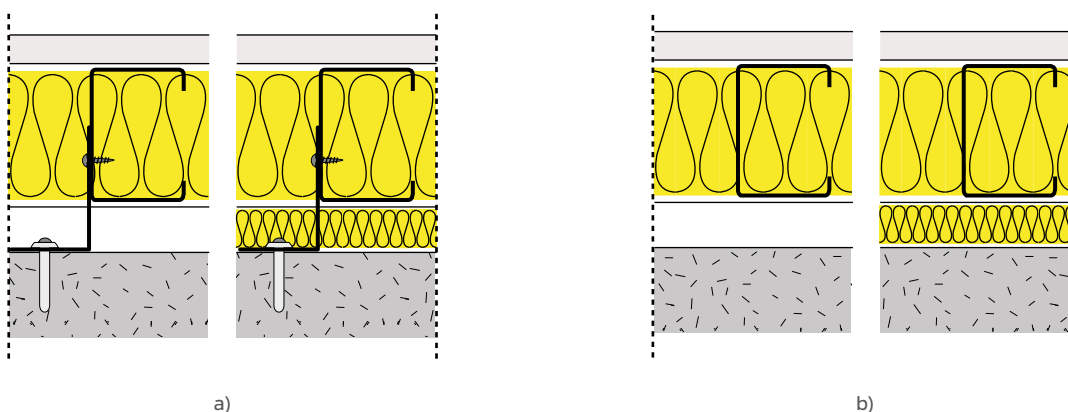
Figura 27: Revestimentos autoportantes: a) fixo pontualmente ao elemento de suporte, b) livre - estrutura independente.
