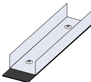
Figura 52: Aplicação de banda acústica entre o perfil raia e o suporte.
