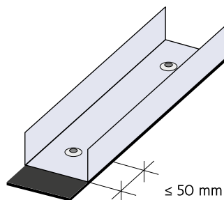
Figura 54: Distância da fixação de extremidade ao topo do perfil raia.
