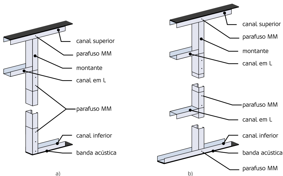
Figura 75: Estrutura metálica em: a) portas; b) janelas.
