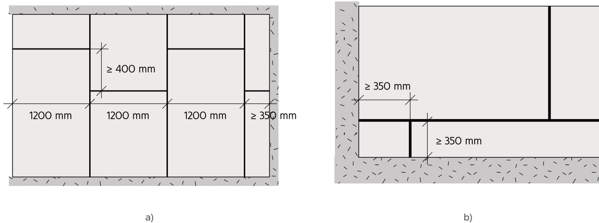
Figura 43: Dimensão mínima admissível das placas e desfasamento das juntas transversais das placas: a) em divisórias e revestimentos; b) em tetos
