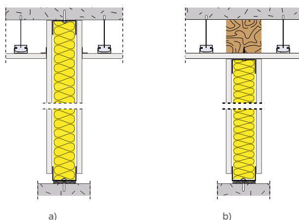
Figura 51: Aplicação do perfil raia superior: a) diretamente na laje; b) sob teto contínuo de placas de gesso.
