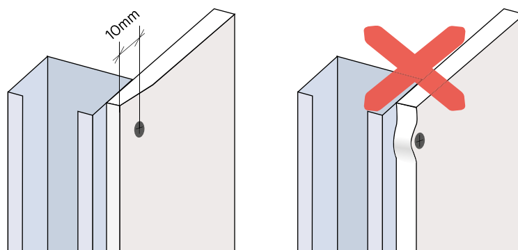
Figura 40: Distância mínima das fixações em relação ao bordo longitudinal.
