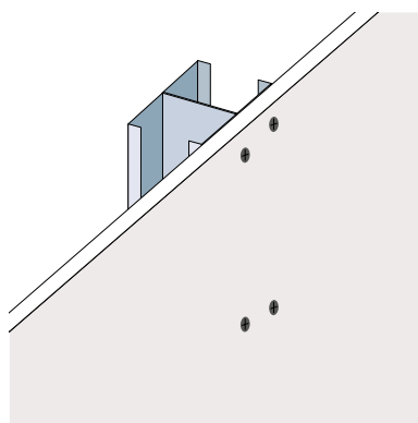
Figura 137: Fixação da placa a perfis montante duplos em “H”.
