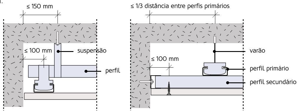
Figura 163: Distância dos perfis da estrutura primária relativamente às paredes periféricas.
