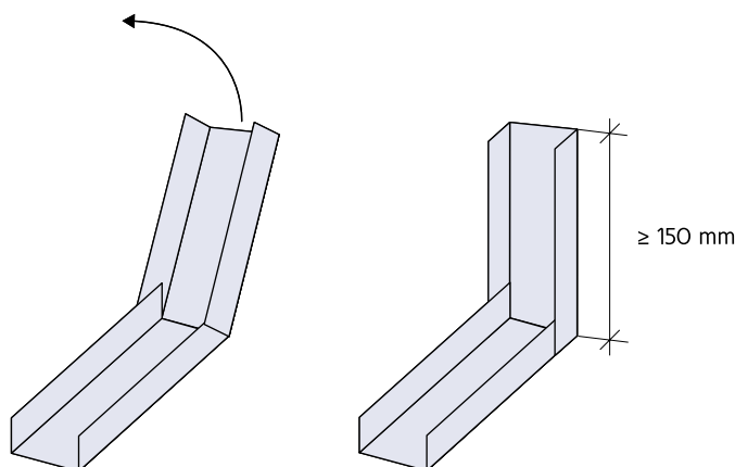
Figura 115: Quinagem dos perfis raia em zonas de aberturas.
