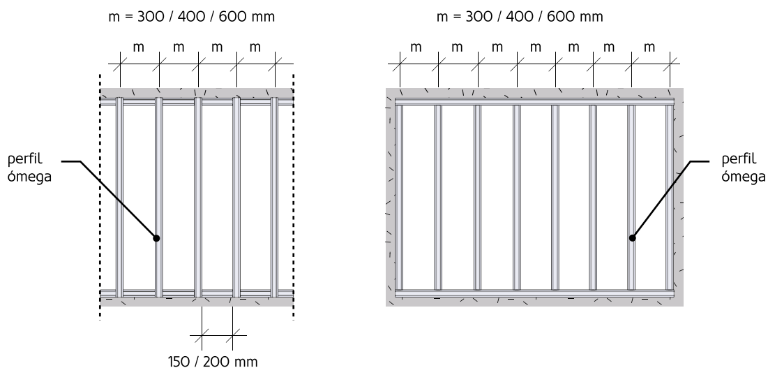
Figura 97: Aplicação de peças de topo.
