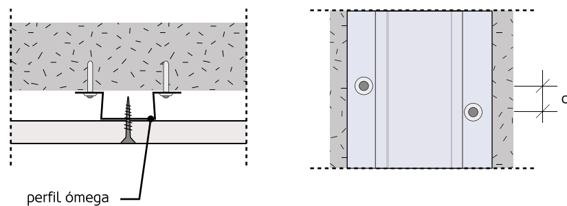
Figura 142: Fixações em perfis ómega.
