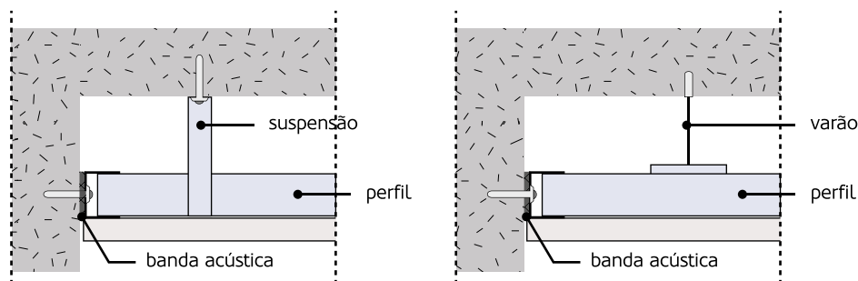
Figura 153: Aplicação de banda acústica entre o suporte e o perfil perimetral.
