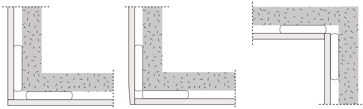
Figura 90: Reforço da colagem em cantos.
