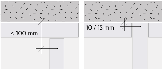
Figura 146: Distância do primeiro parafuso em relação à parede periférica.
