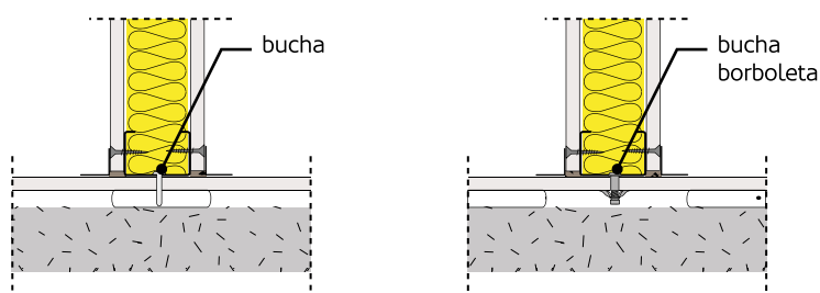
Figura 91: Reforço da colagem em encontros.
