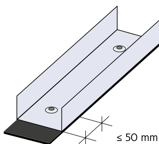
Figura 111: Distância da fixação de extremidade ao topo do perfil raia.
