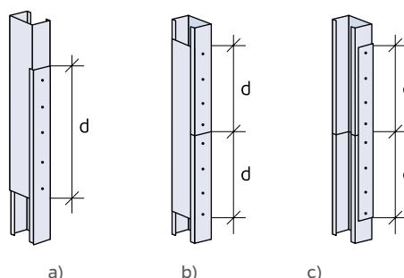
Figura 61: Emendas possíveis em perfis montante:
