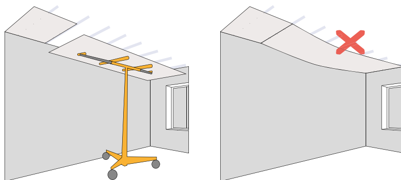
Figura 165: Fixação das placas de gesso em tetos contínuos.
