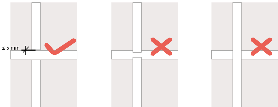
Figura 167: Aplicação de bandas de papel.
