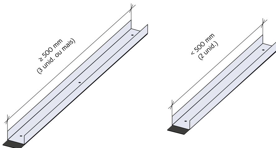
Figura 56: Número de fixações em função do comprimento do perfil.
