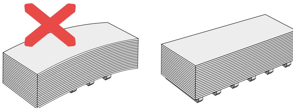
Figura 18: Colocação das placas sobre calços.
