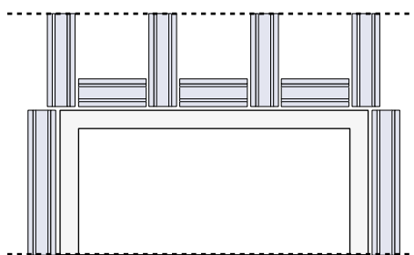
Figura 100: Aplicação da estrutura no limite de aberturas.
