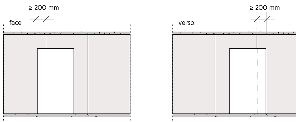
Figura 85: Contorno de vãos em divisórias.
