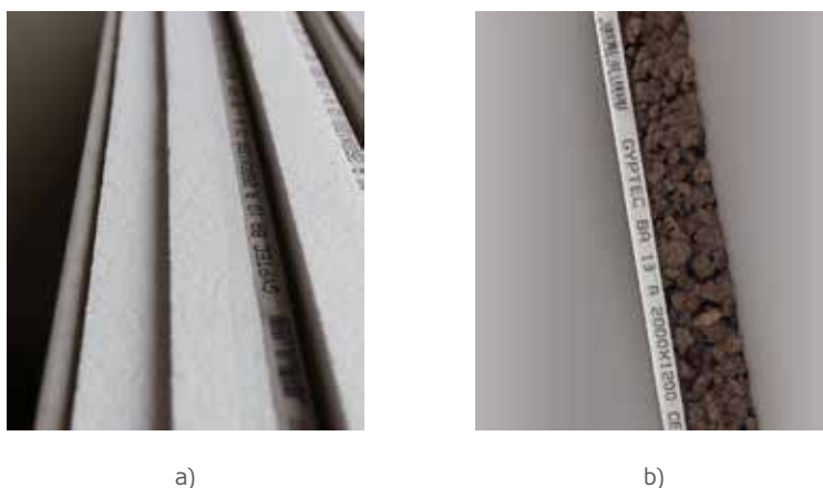
Figura 8: Tipos de placas compostas: a) com EPS, b) com ICB.
