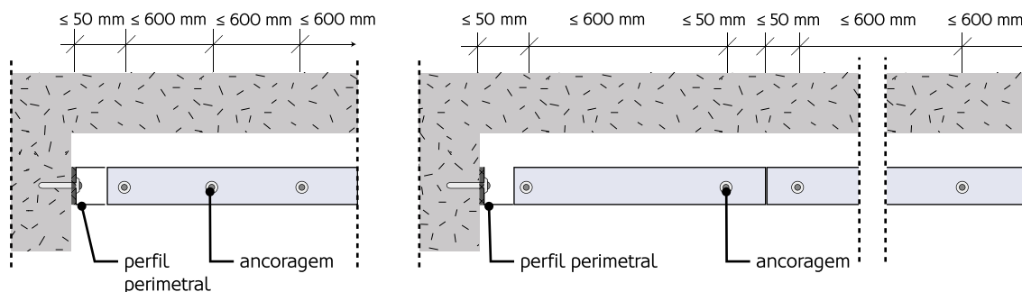
Figura 151: Fixação dos perfis perimetrais.
