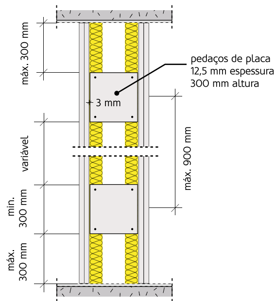
Figura 70: Ligação entre estruturas.
