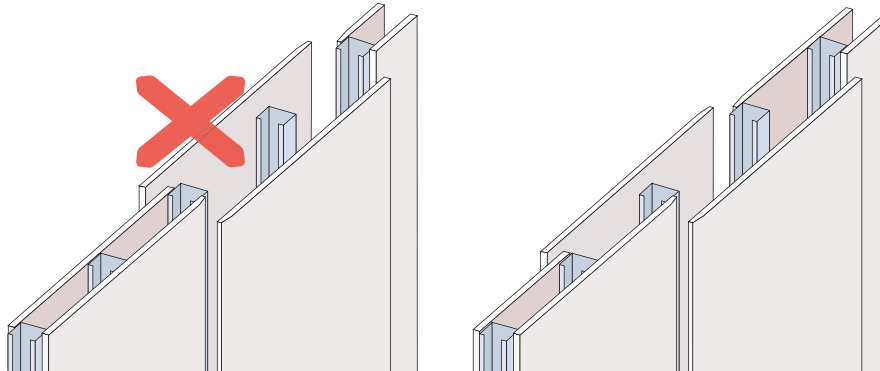
Figura 79: Juntas longitudinais em divisórias de placa simples.
