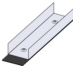
Figura 109: Aplicação de banda acústica entre o perfil raia e o suporte.
