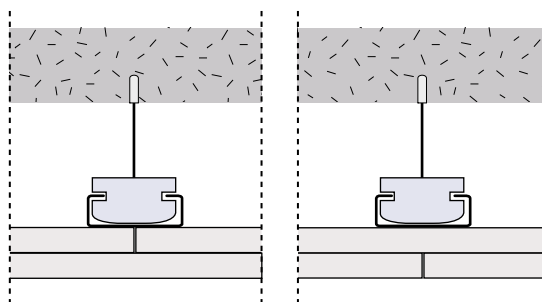
Figura 159: Desfasamento de juntas em tetos de placa dupla ou múltipla.
