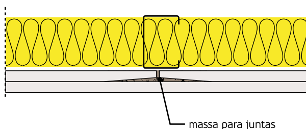
Figura 166: Tratamento de juntas em sistemas de placa dupla ou múltipla.
