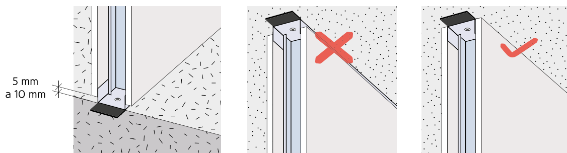
Figura 77: Aplicação das placas encostadas ao teto e afastadas 10 mm do pavimento.
