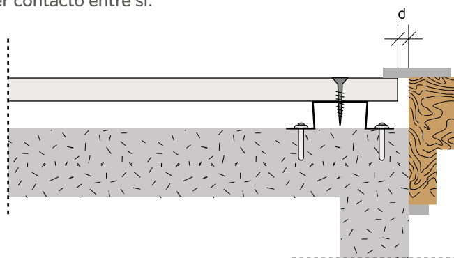
Figura 108: Aplicação das placas no limite da abertura.
