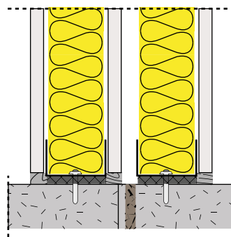
Figura 47: Junta ao longo do eixo da divisória.
