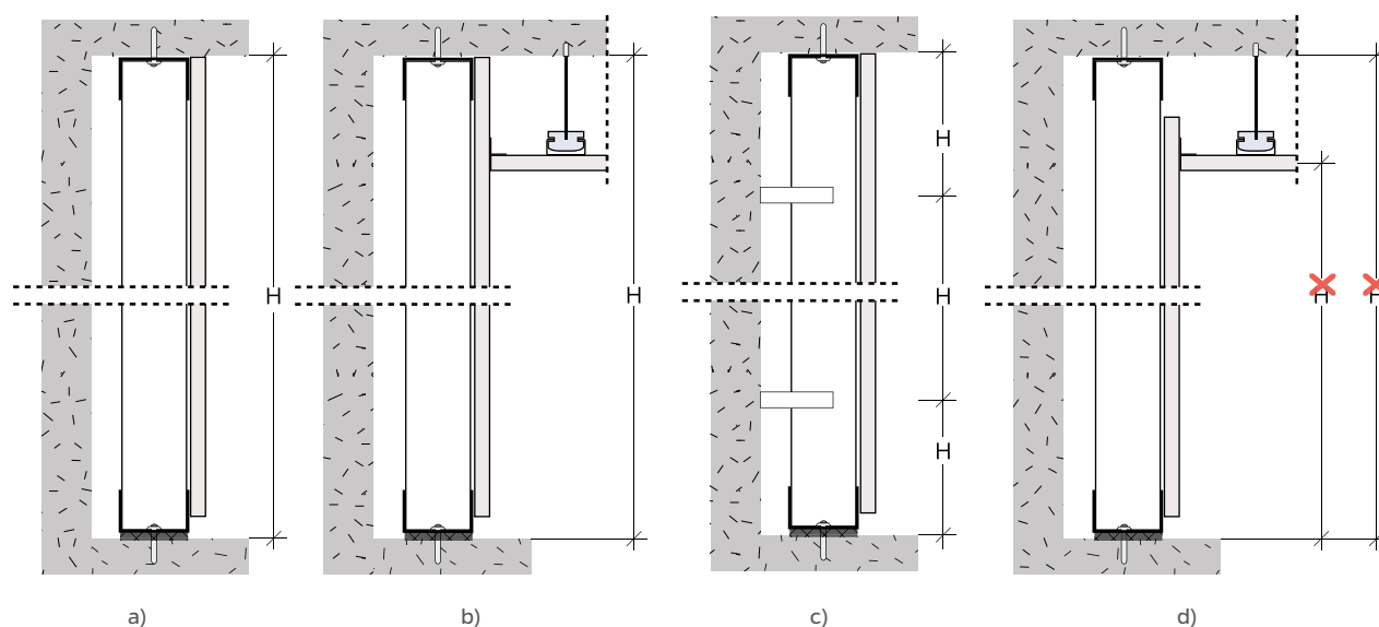
Figura 29: Condições a observar na determinação das alturas máximas.
