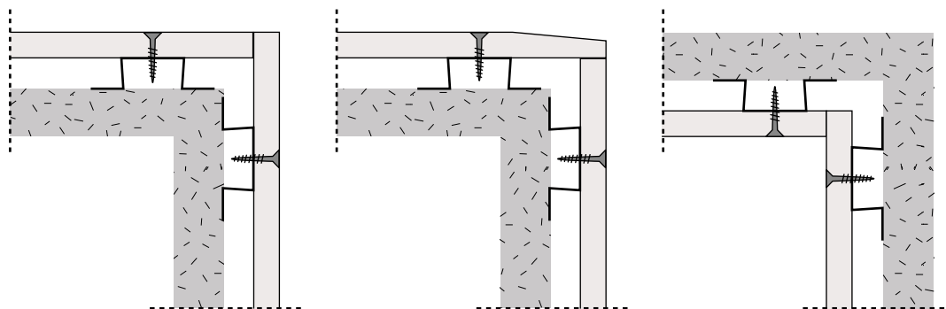
Figura 98: Reforço da estrutura metálica em cantos.
