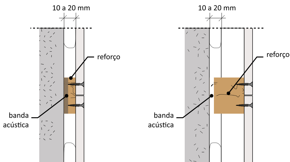
Figura 28: Reforços em revestimentos diretos com cola adesiva.
