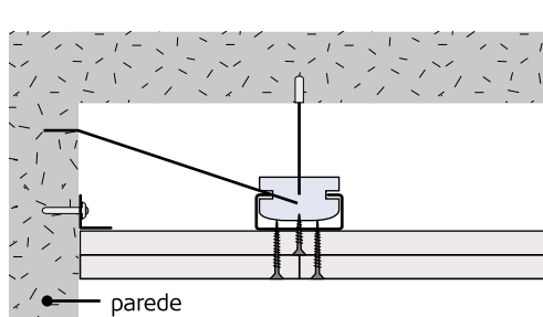
Figura 34: Tensores de reforço.
