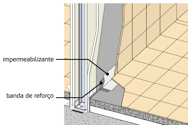
Figura 36: Reforço do perímetro do compartimento com impermeabilizantes e bandas de reforço.
