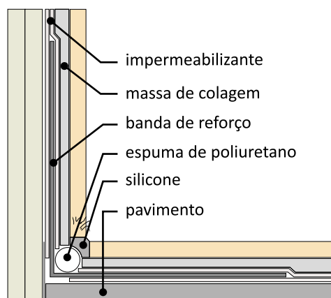
Figura 37: Reforço do sistema de impermeabilização no perímetro inferior do compartimento e cantos ou encontros verticais.
