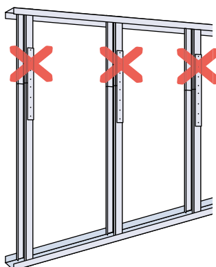
Figura 62: Alinhamento de emendas em perfis montante.
