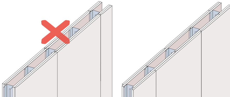
Figura 80: Juntas longitudinais em divisórias de placa dupla.
