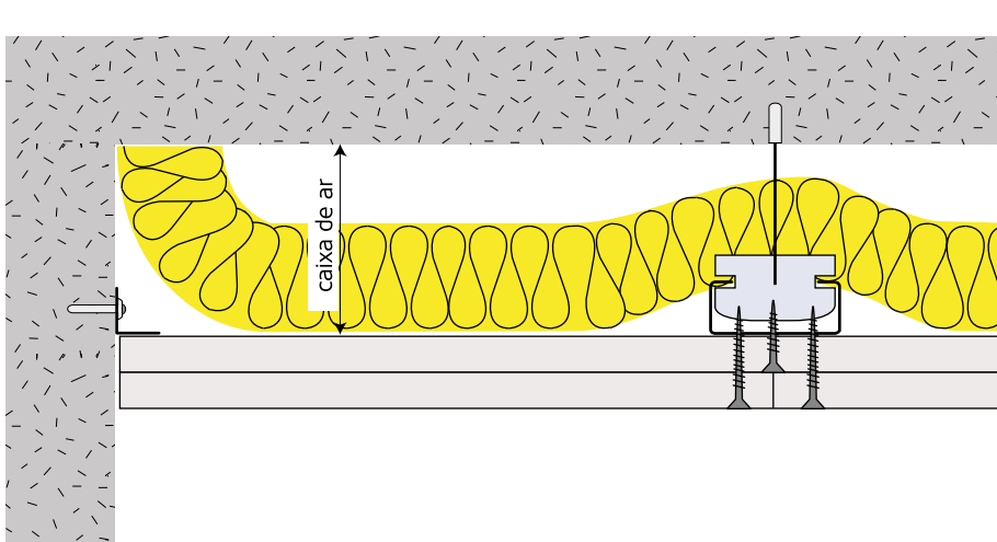
Figura 49: Isolamento no interior da caixa-de-ar de tetos contínuos.
