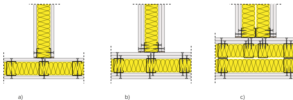
Figura 72: Ligações em encontros em T: a) Estrutura simples – placa simples; b) Estrutura simples – placa dupla; c) Estrutura dupla – placa dupla.
