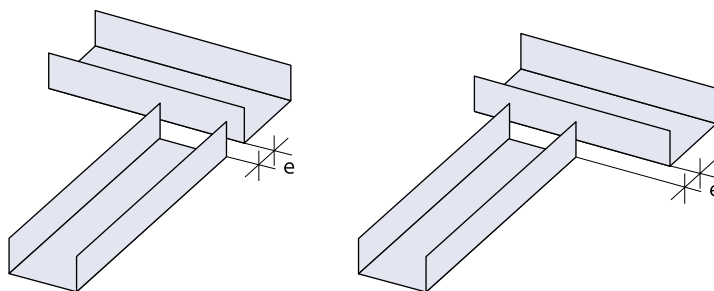
Figura 114: Afastamento entre perfis raia de divisórias que se intersectam.
