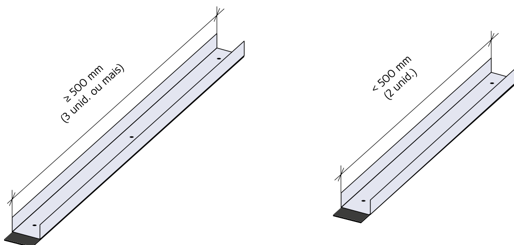
Figura 112: Número de fixações em função do comprimento do perfil.
