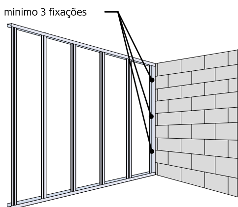
Figura 119: Fixação mínima.
