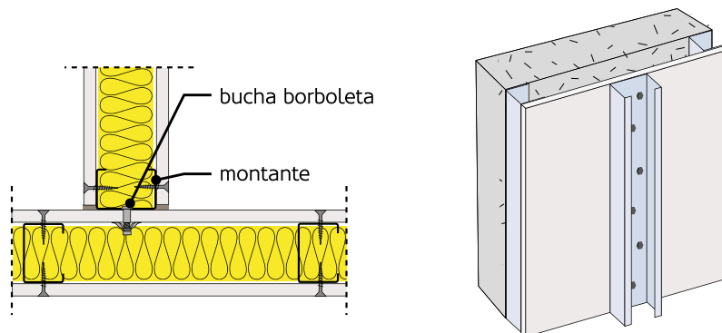
Figura 129: Ligação de um perfil montante de arranque a um sistema existente.
