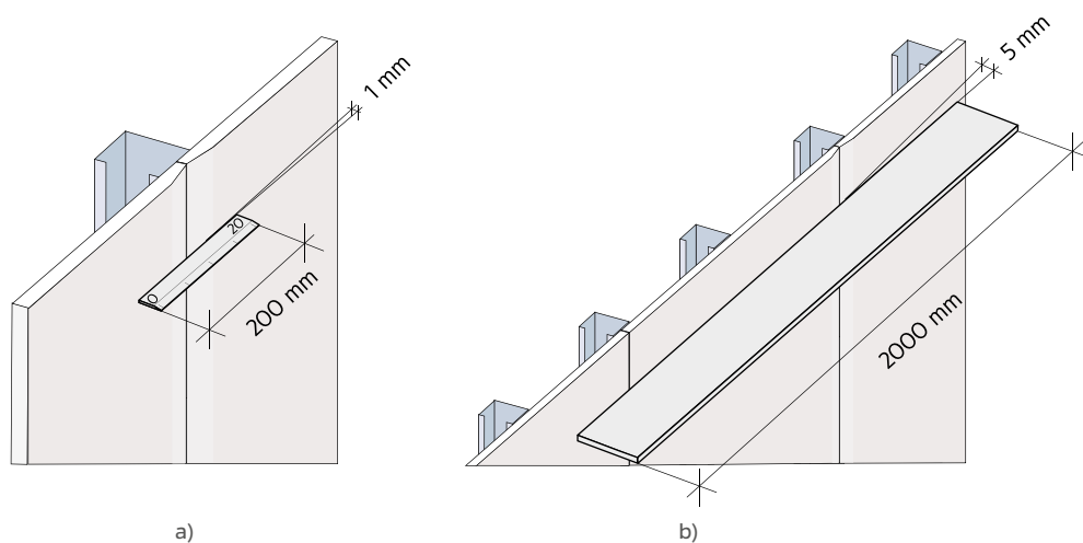
Figura 169: Verificação da planeza: a) localizada; b) geral.
