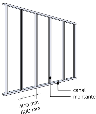
Figura 123: Afastamento entre perfis montante.
