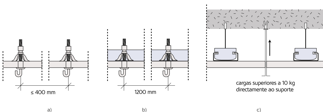
Figura 173: Tipos de fixação:
