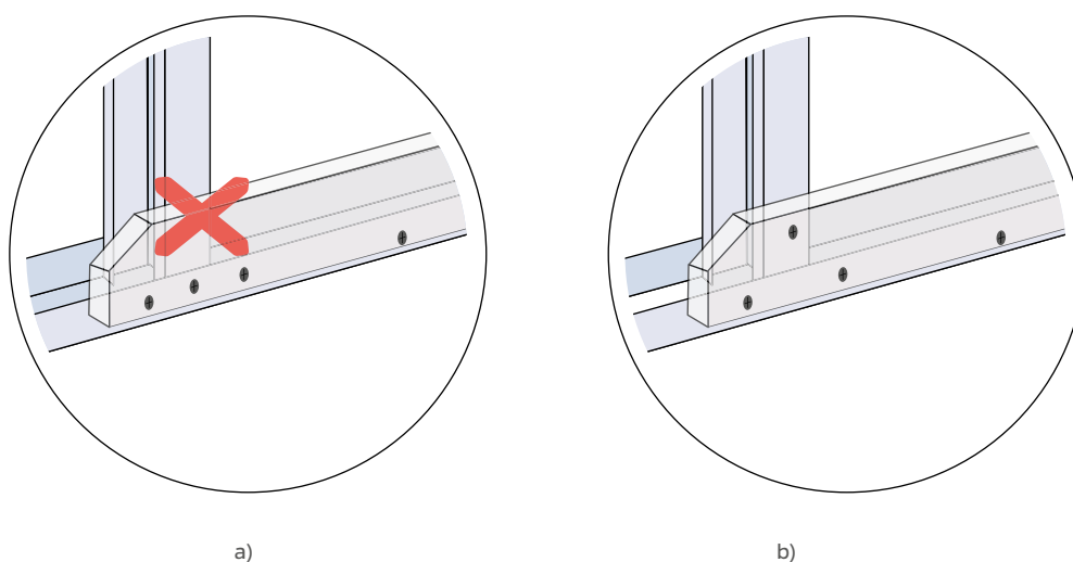
Figura 83: a) Fixação simultânea entre placa, perfil montante e perfil raia; b) Fixação da placa ao perfil raia e da placa ao perfil montante, separadamente.
