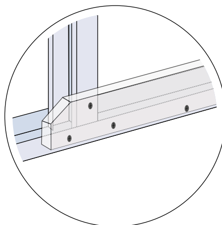
Figura 136: Fixação da placa ao perfil raia e da placa ao perfil montante, separadamente.
