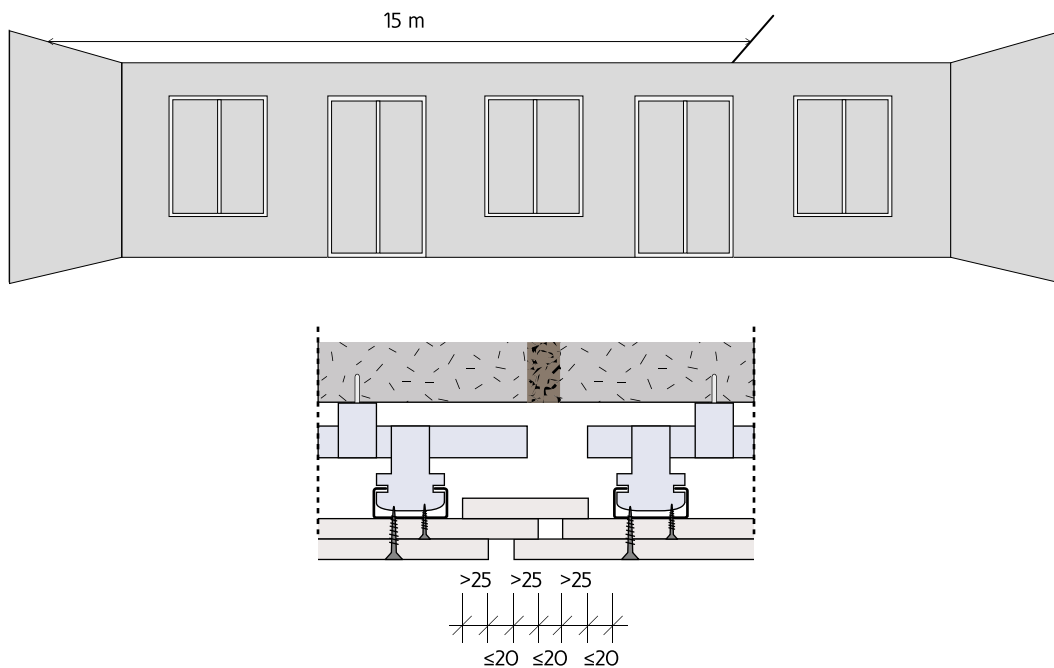
Figura 35: Juntas de dilatação.
