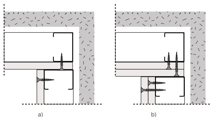
Figura 127: Ligações em cantos reentrantes:
