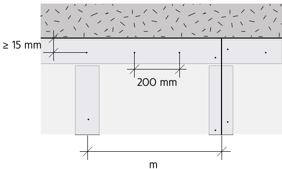
Figura 147: Fixação das placas a perfis perimetrais contínuos.
