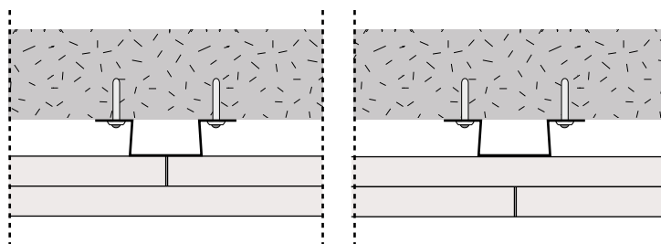
Figura 145: Desfasamento de juntas em tetos de placa dupla ou múltipla.
