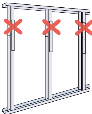
Figura 118: Alinhamento de emendas em perfis montante.
