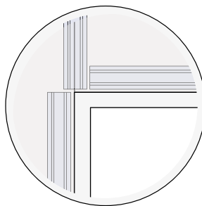
Figura 107: Aplicação da estrutura no limite de aberturas.
