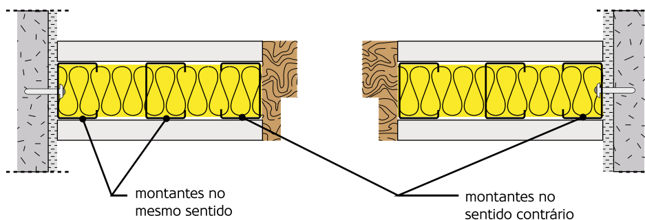
Figura 124: Posição dos perfis montante.
