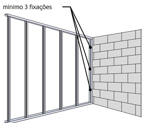
Figura 63: Fixação mínima de perfis montante de extremidade.
