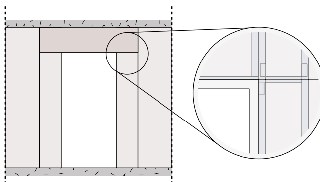
Figura 86: Contorno de vãos em divisórias.
