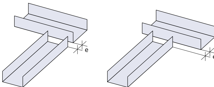
Figura 58: Afastamento entre perfis raia de divisórias que se intersectam.
