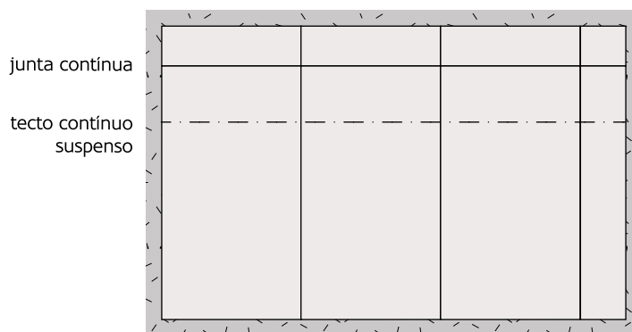
Figura 133: Alinhamento de juntas transversais.
