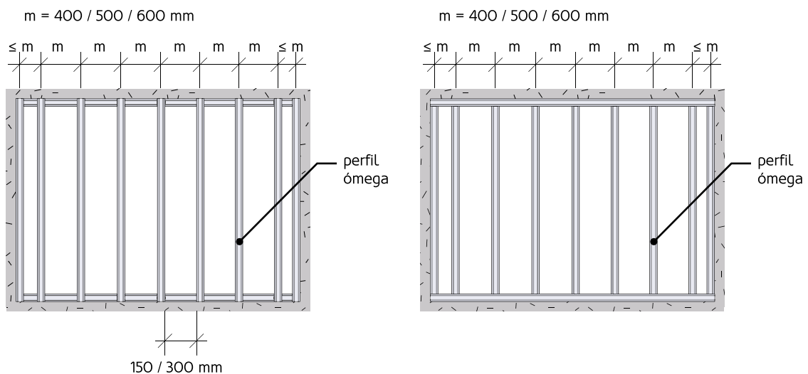
Figura 143: Aplicação de perfis de remate.
