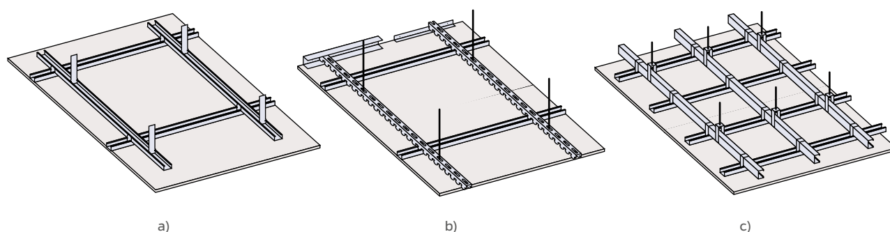
Figura 32: Tetos contínuos suspensos de estrutura composta: a) com perfis teto, b) com régua de suspensão, c) com perfis montante.
