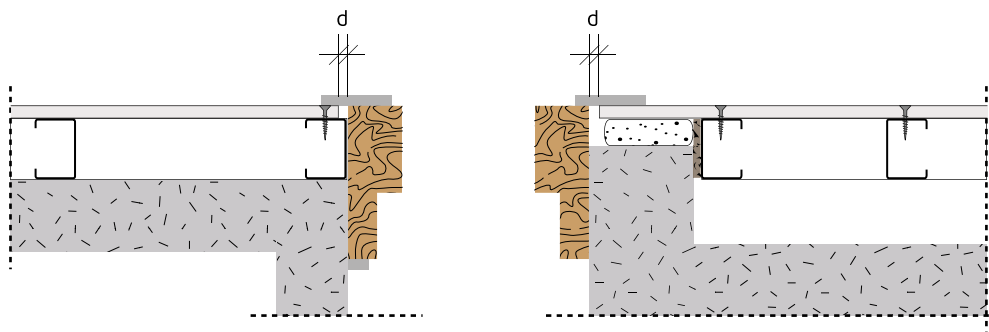
Figura 140: Aplicação das placas no limite da abertura.
