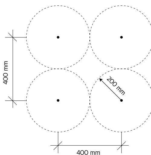
Figura 171: Distância máxima entre fixações.
