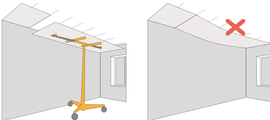
Figura 144: Fixação das placas de gesso em tetos contínuos.
