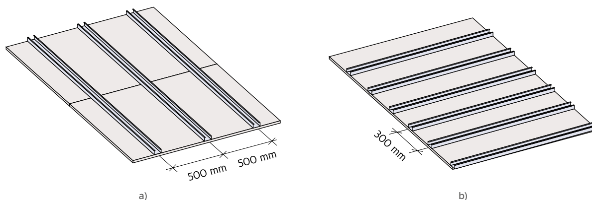
Figura 33: Distância entre perfis: a) aplicação das placas perpendicularmente aos perfis, b) aplicação das placas paralelamente aos perfis.
