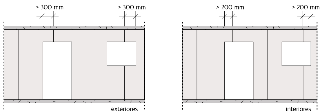
Figura 105: Contorno de vãos em revestimentos diretos com perfis ômega.
