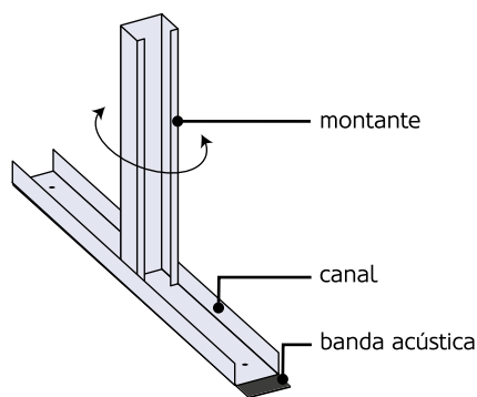
Figura 65: Encaixe dos perfis montante nos perfis raia.
