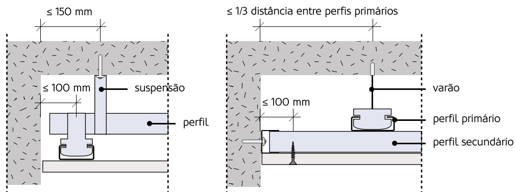
Figura 160: Distância dos pendurais e suspensões da estrutura primária relativamente às paredes periféricas.
