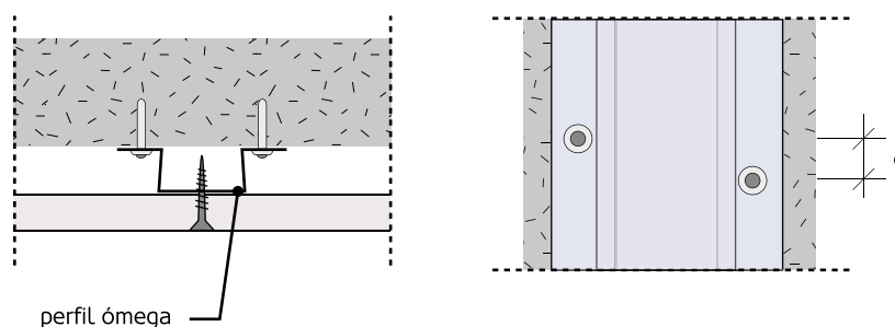
Figura 96: Fixações em perfis ómega.
