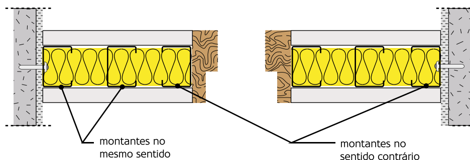
Figura 68: Posição dos perfis montante.
