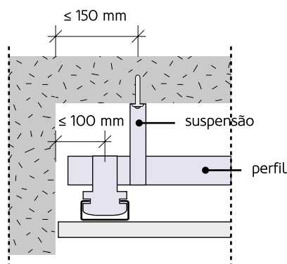
Figura 164: Distância dos perfis da estrutura secundária relativamente às paredes periféricas.
