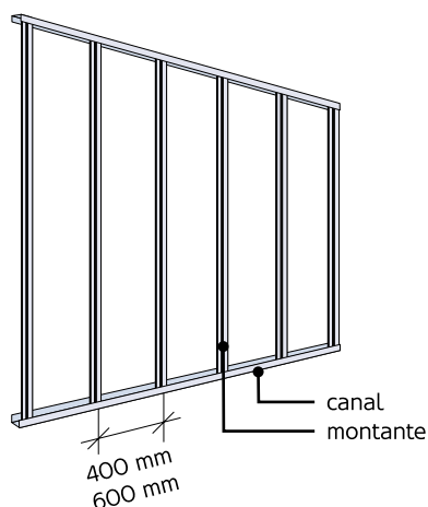
Figura 67: Afastamento entre perfis montante.
