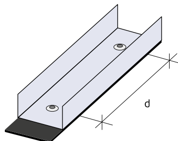
Figura 110: Afastamento entre fixações.
