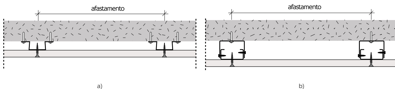
Figura 30: Tetos contínuos diretos: a) com perfis ómega, b) com perfis de teto.
