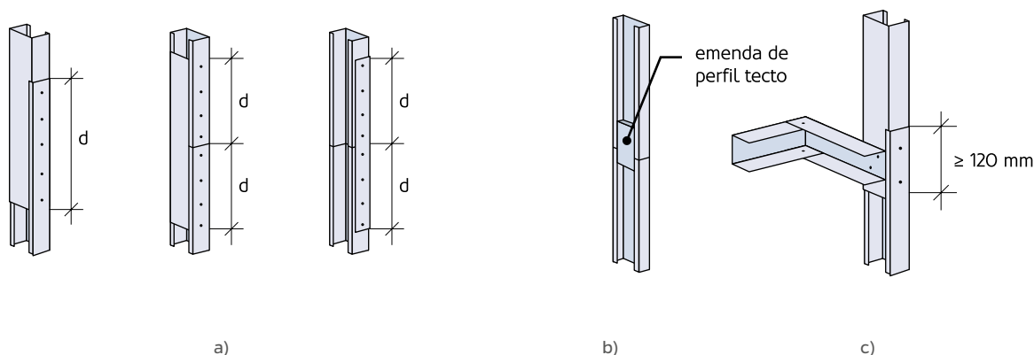
Figura 117: Emendas possíveis em elementos verticais:
