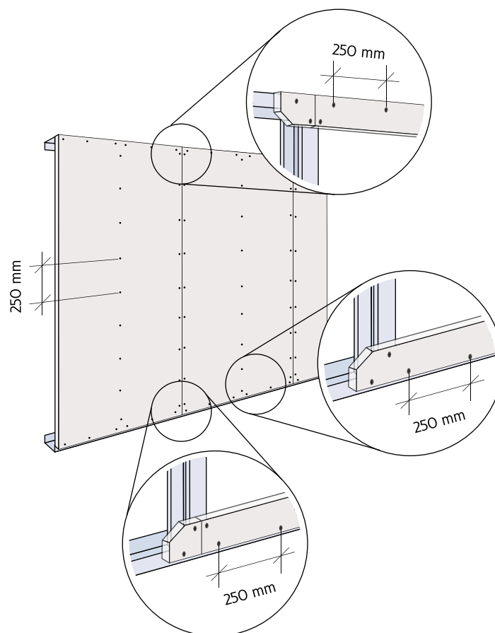
Figura 82: Afastamento entre fixações das placas aos perfis raia.
