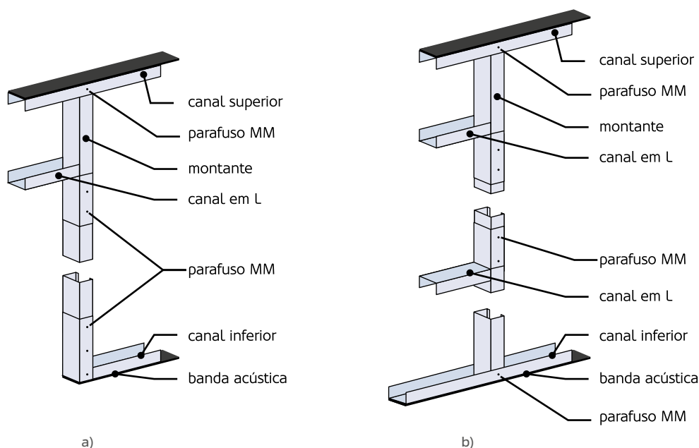
Figura 131: Estrutura metálica em: a) portas; b) janelas.
