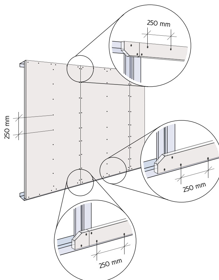
Figura 135: Afastamento entre fixações das placas aos perfis raia.
