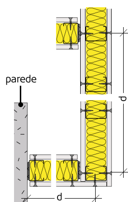
Figura 24: Comprimentos livres máximos.
