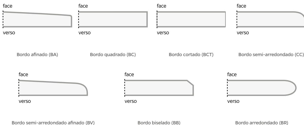
Figura 7: Tipos de bordos das placas de gesso laminado.
