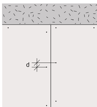
Figura 42: Fixações no bordo longitudinal de duas placas contíguas.
