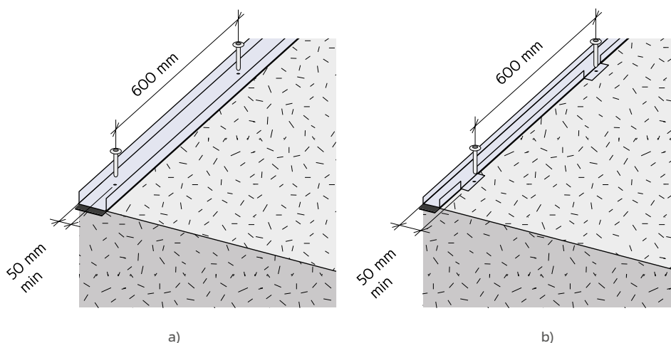
Figura 55: Fixação do perfil raia na extremidade de uma laje: a) perfis de 70 mm e 90 mm; b) perfil de 48 mm.
