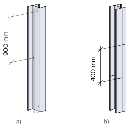
Figura 122: Ligação entre dois perfis montante: a) parafusos em quincôncio; b) juntas em perfis montante em “H”.
