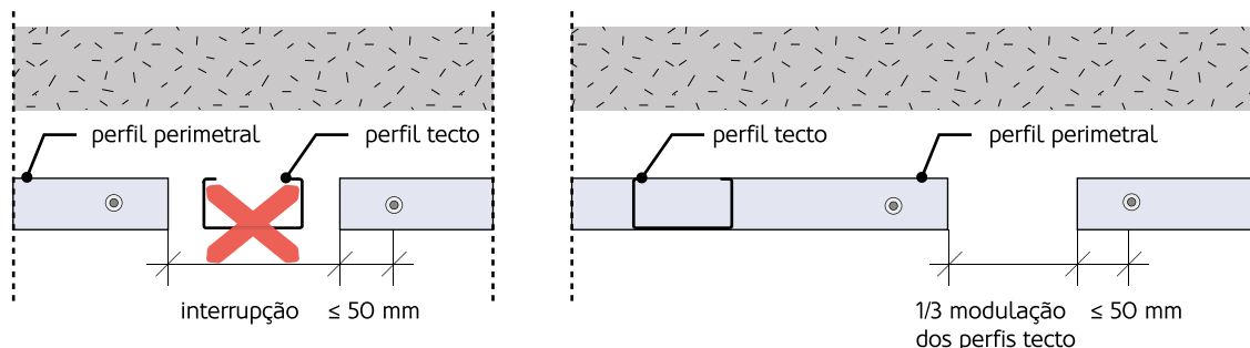
Figura 152: Interrupção dos perfis perimetrais.
