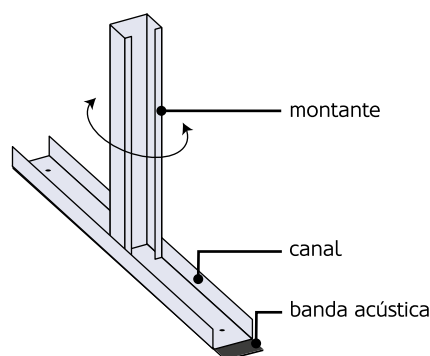
Figura 121: Encaixe dos perfis montante nos perfis raia.
