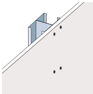
Figura 84: Fixação da placa a perfis montante duplos em “H”.
