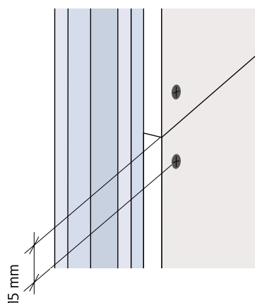
Figura 41: Distância mínima das fixações em relação ao bordo transversal.
