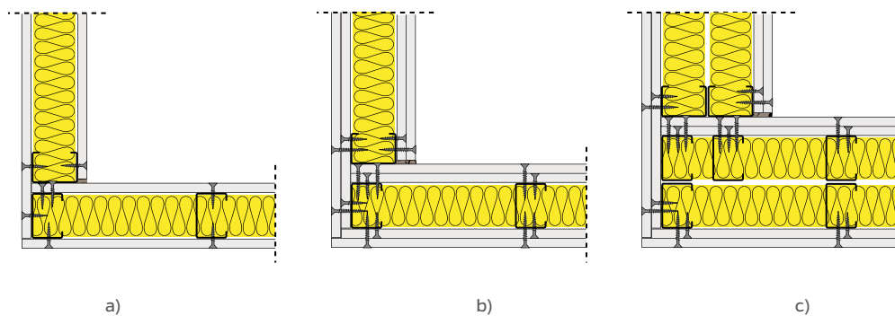
Figura 71: Ligações em cantos: a) Estrutura simples - placa simples; b) Estrutura simples - placa dupla; c) Estrutura dupla - placa dupla.
