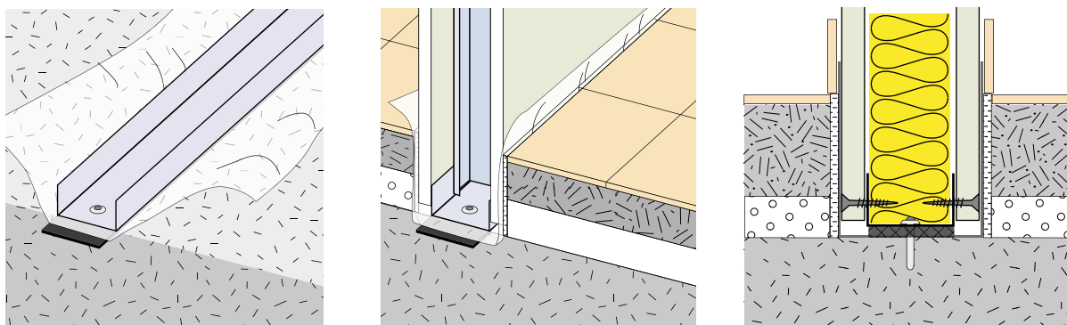
Figura 50: Aplicação de película de polietileno, entre a laje de betão e o perfil raia, e de tiras de material flexível, para separação da divisória do enchimento da laje.
