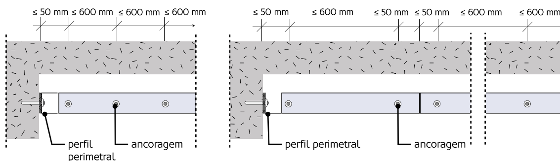
Figura 161: Fixação dos perfis perimetrais.
