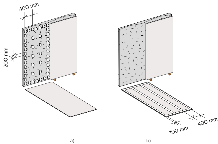
Figura 89: Aplicação da cola: a) por pontos; b) em tiras.
