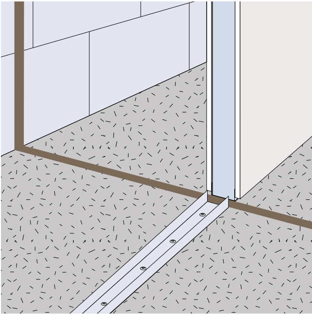
Figura 25: Junta de dilatação do edifício.
