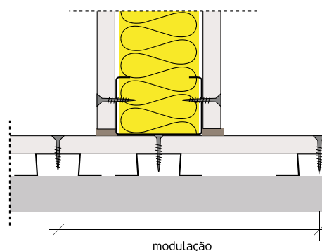
Figura 99: Reforço da estrutura metálica em encontros.
