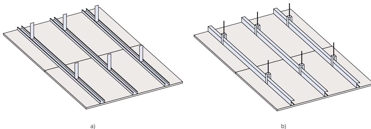
Figura 31: Tetos contínuos suspensos de estrutura simples: a) com perfis teto, b) com perfis montante.
