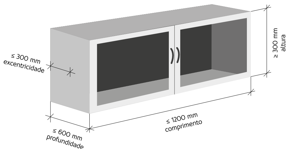
Figura 172: Cargas excêntricas.
