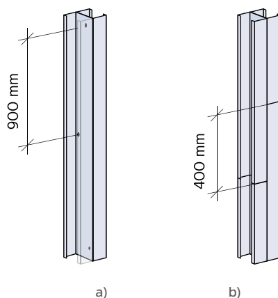
Figura 66: Ligação entre dois perfis montante: a) parafusos em quincôncio; b) juntas em perfis montante em “H”.
