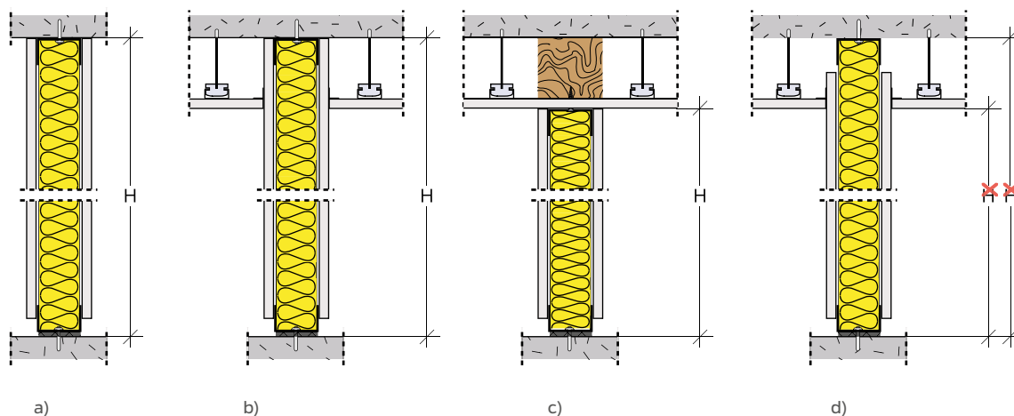
Figura 23: Condições a observar na determinação das alturas máximas.
