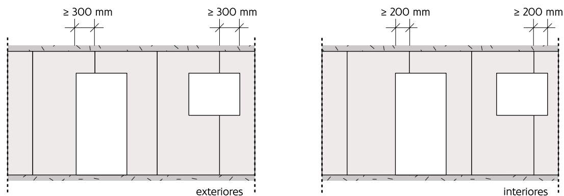
Figura 93: Contorno de vãos em revestimentos diretos com cola adesiva.
