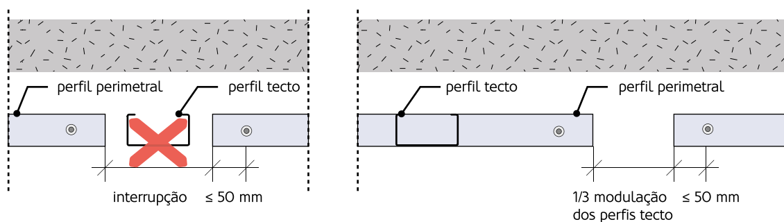
Figura 162: Interrupção dos perfis perimetrais.
