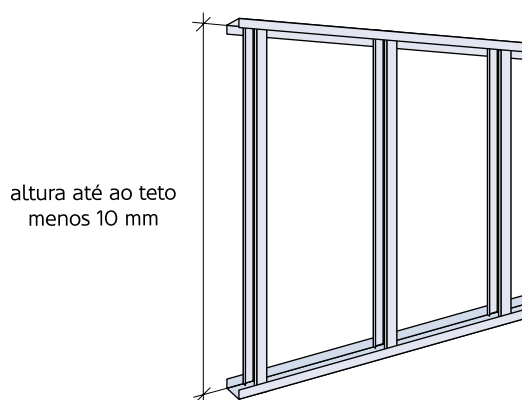
Figura 116: Comprimento dos montantes.
