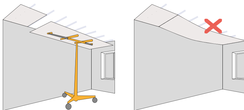
Figura 158: Fixação das placas de gesso em tetos contínuos.
