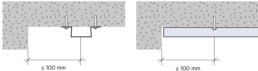
Figura 141: Afastamento máximo dos perfis relativamente às paredes periféricas.
