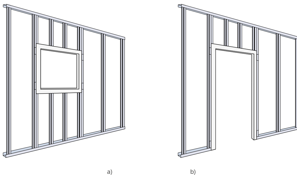
Figura 132: Estrutura metálica em: a) janelas; b) portas.
