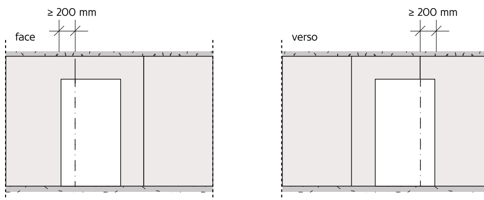
Figura 138: Contorno de vãos em revestimentos autoportantes.
