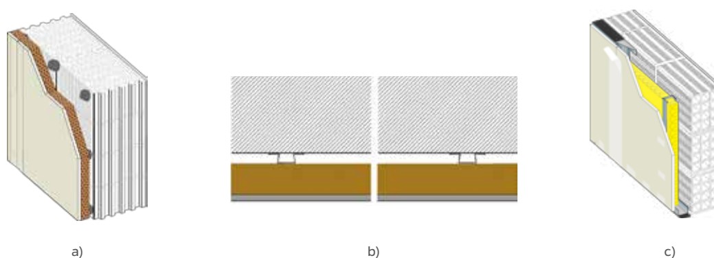
Figura 26: Tipos de revestimentos: a) direto com cola adesiva, b) direto com estrutura auxiliar, c) autoportante.
