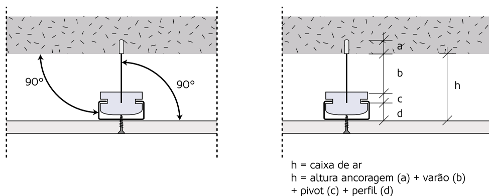
Figura 149: Aplicação de pendurais.
