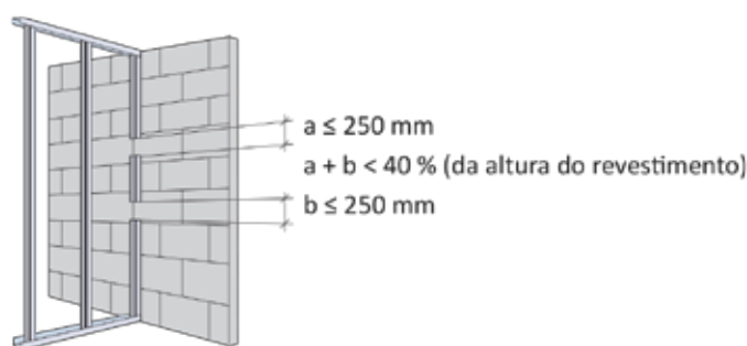
Figura 120: Interrupções permitidas nos perfis montante de extremidade.
