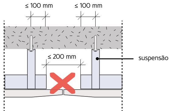
Figura 155: Juntas de placas na zona de interrupção de perfis.
