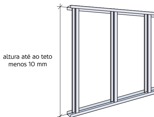
Figura 60: Comprimento dos perfis montante.
