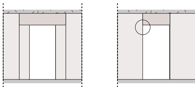
Figura 106: Contorno de vãos em revestimentos diretos com perfis ômega.
