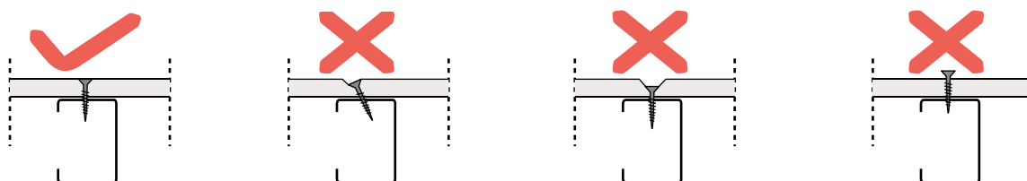
Figura 39: Perpendicularidade dos parafusos e respetiva penetração na placa.
