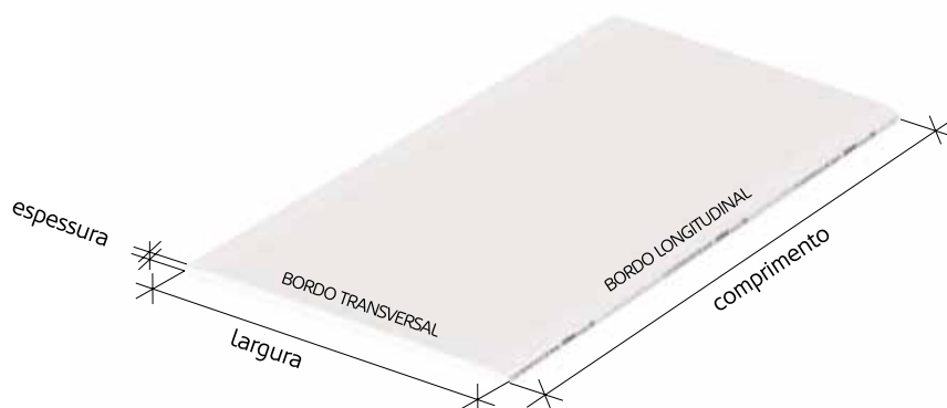
Figura 6: Dimensões das placas de gesso laminado.
