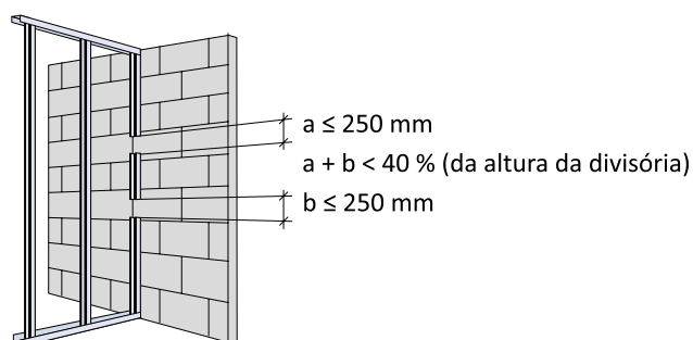
Figura 64: Interrupções permitidas nos perfis montante de extremidade.
