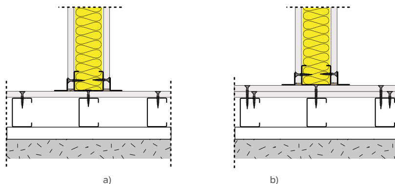
Figura 128: Ligações em encontros: a) Placa simples; b) Placa dupla.
