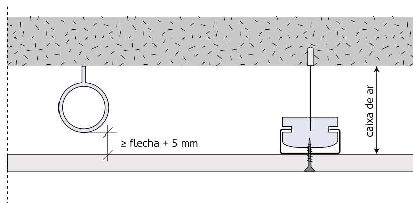
Figura 48: Altura da caixa-de-ar quando há instalações no interior do teto.
