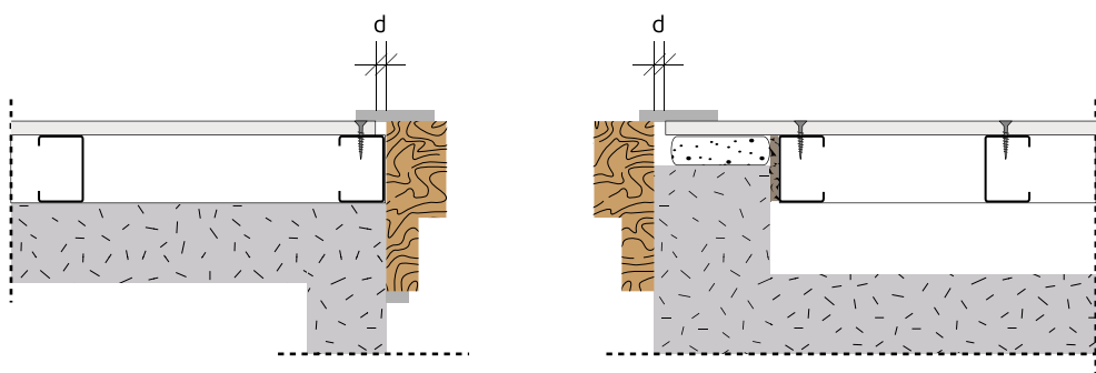
Figura 130: Aplicação de elementos construtivos que definem as aberturas.
