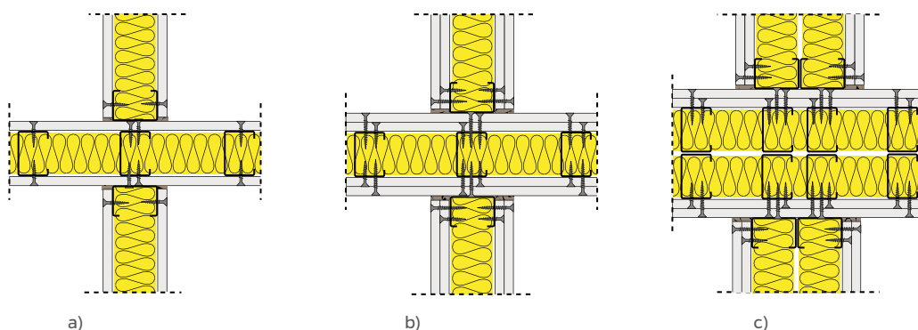
Figura 73: Ligações em encontros em cruz: a) Estrutura simples – placa simples; b) Estrutura simples – placa dupla; c) Estrutura dupla – placa dupla.
