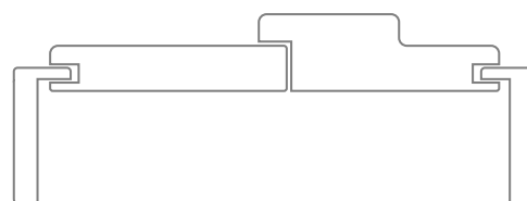
Esquema solución especial Special request frame section
